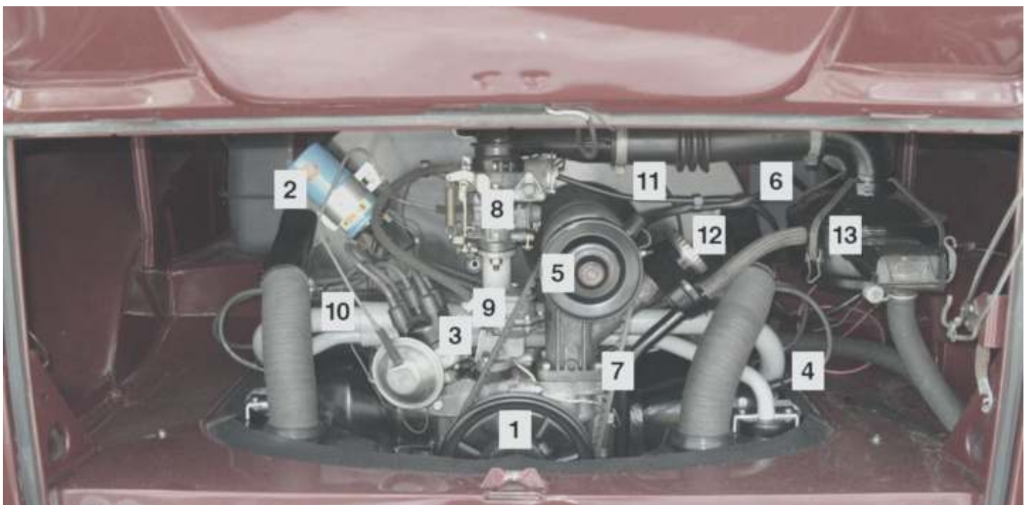
Un motor (casi) vertical 1600 tipo 1 de uno de los primeros autobuses con ventana
